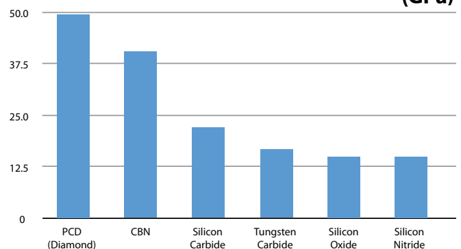
Hardness (Knoop)
